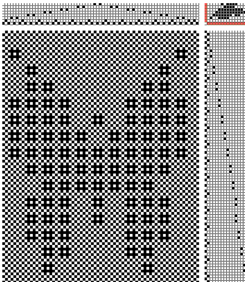
Figuur 9 – werktekening vlinder in kettingflotteringen
